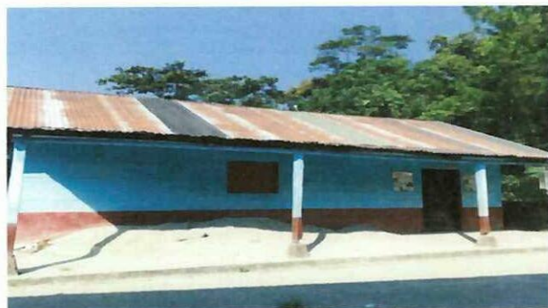
Foto 4: Sustrucción de cubierta de lámina en aula debido a mal estado y sustrucción de estructura de madera por estructura metálica en techo.
